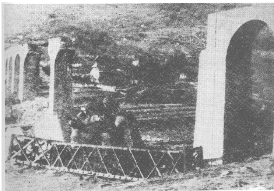
Vijadukt Bender (Knin) nakon rušenja 1943. godine
