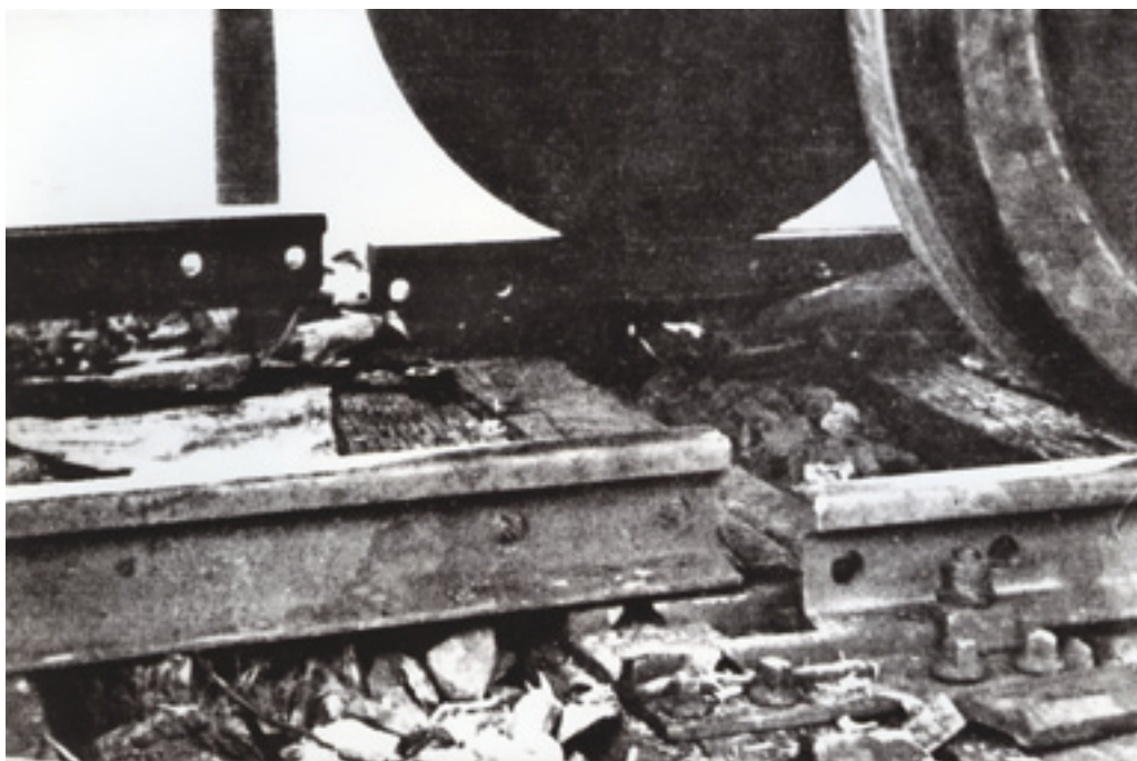
33. Tako razmaknjeni tirnici sta povzročili iztirjenje vlaka.
