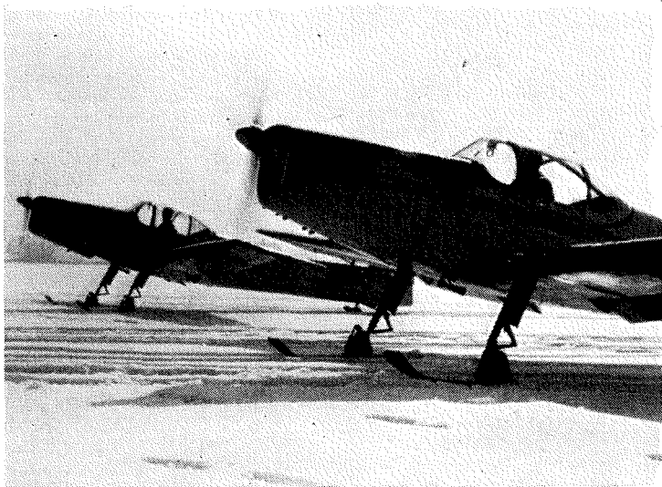
Športno-turistični letali KB-6 »Matajur« na smučeh
