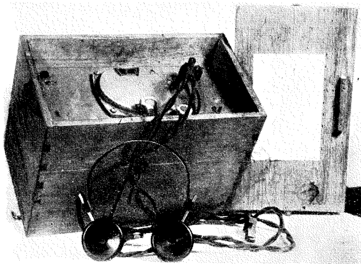
Radijski sprejemnik ob baterijah, ki ga je uporabljal med NOV dr. Marijan Breclj
