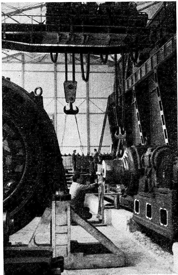
Notranjost motorne hale nove valjarne na Javorniku za časa gradnje
