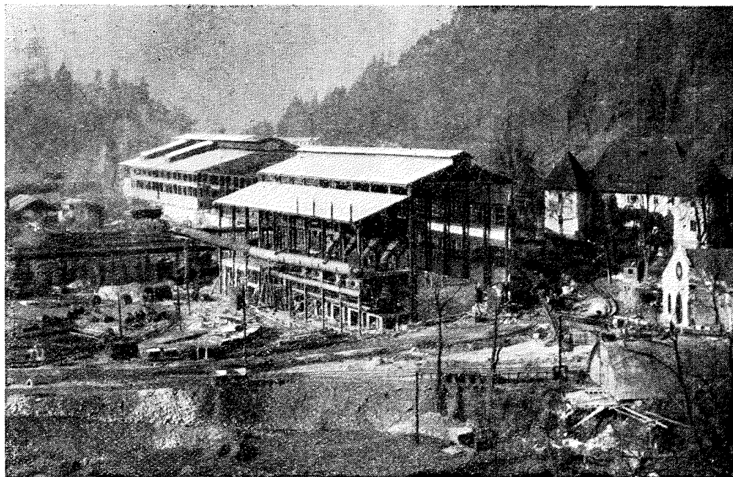
Pogled na novo veliko valjarno debele pločevine na Javorniku. Desno fuži narski Zoisov gradič
