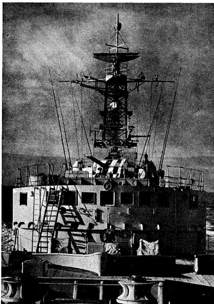
Fotografija nam prikazuje komanđni most in prednji jadrnik protipodmorniške fregate »Relentless«. To je prva angleška vojna ladja, izdelana iz posebnega materiala, ki je odporen proti učinkom atomskih izstrelkov
