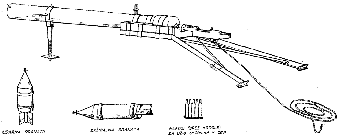
Gornja slika nam prikazuje načrt topa, kakršnega so izdelali junija 1942. leta partizani na Turjaku
