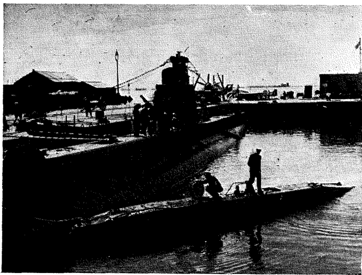
Na sliki: spredaj vidimo angleško podmornico — »prtilikavec« poleg podmornice najmanjše normalne velikosti. Posadko podmornice — »prtilikavca« sestavljajo trije člani in komandant. Podmornica — »prtilikavec« je namenjena specialni podmorniški službi.
