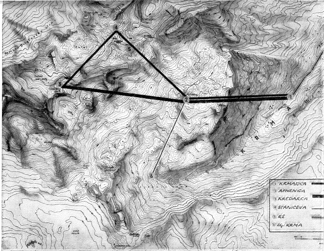
Situacija območja triglavskih žičnic.
